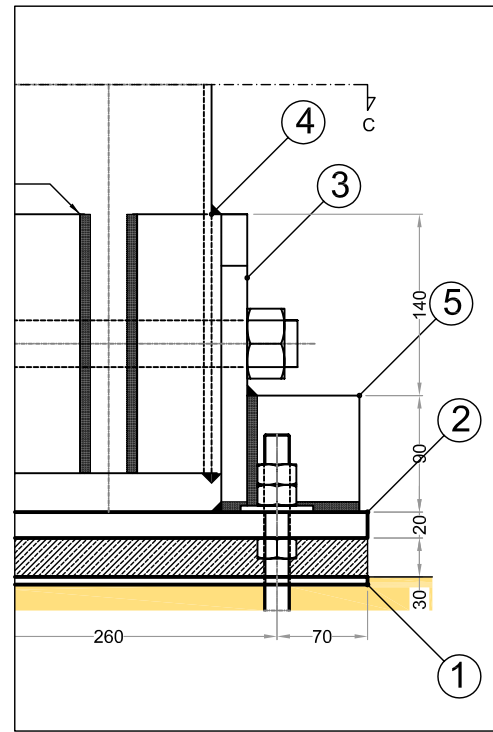
DETTAGLIO ESECUTIVO
