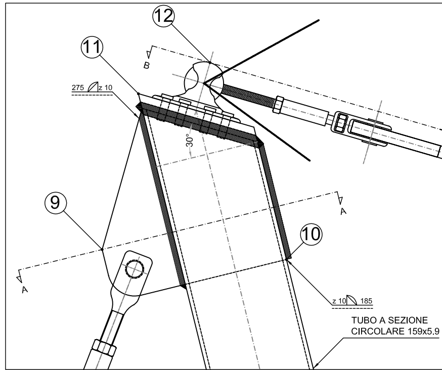
DETTAGLIO ESECUTIVO
