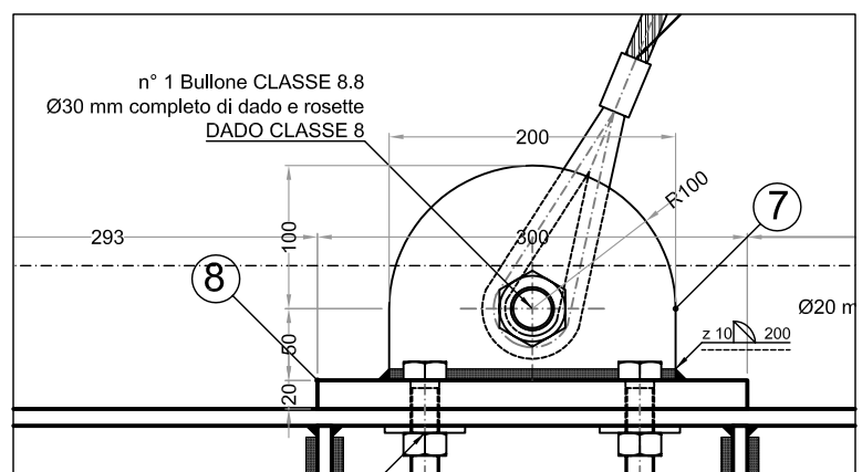
DETTAGLIO ESECUTIVO
