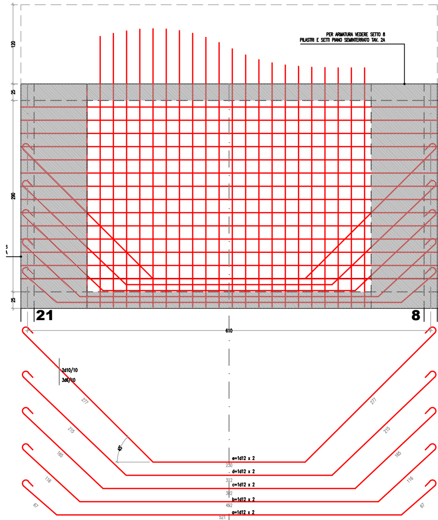
DETTAGLIO ESECUTIVO
