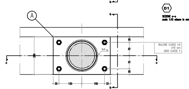
DETTAGLIO
